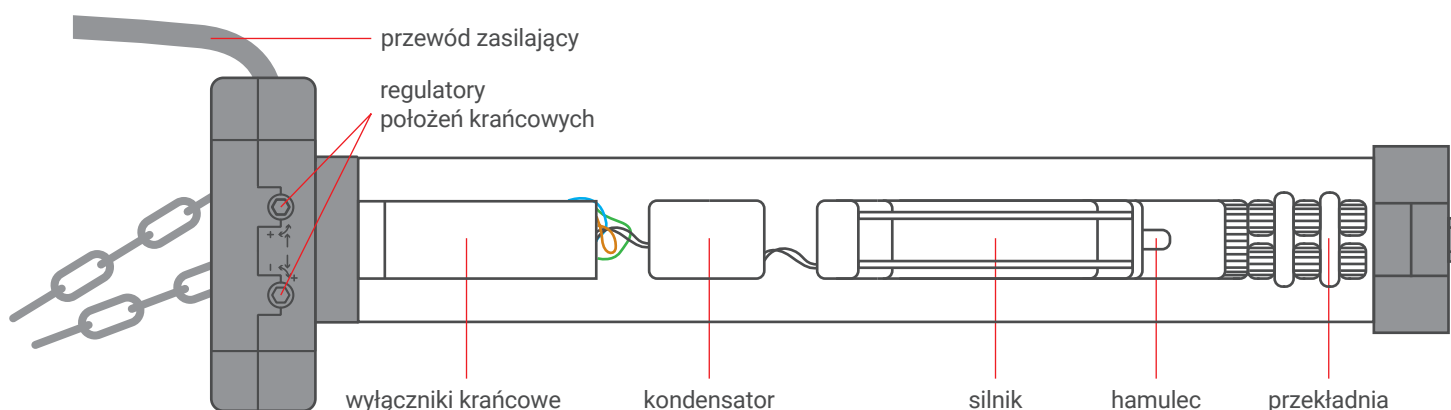
Napęd rurowy 59MB
